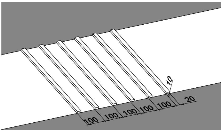
图3 减速带尺寸 (单位: mm)
