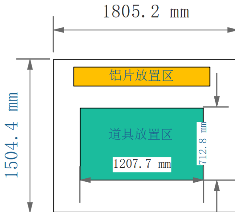
图 1-比赛场地示意
