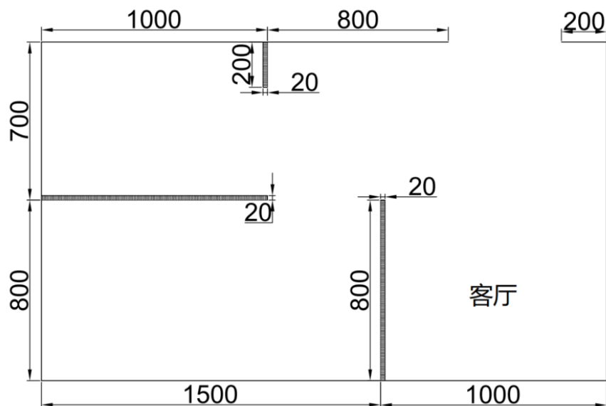
图 2 - 实体机器人场地规格，墙高 10cm
