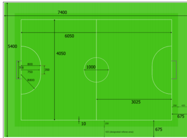
图 1 场地尺寸示意图
